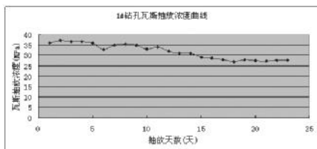
图 3-2 1#孔设计工艺瓦斯抽采浓度曲线图
