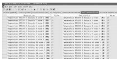
图 3:TP 车各轴温传感器通讯状态
