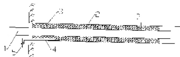
图 2-1 双侧聚氨酯-水泥砂浆封孔示意图
