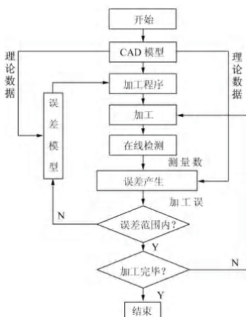
图1 数控加工误差补偿流程
