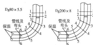
图 2 管线检测图
