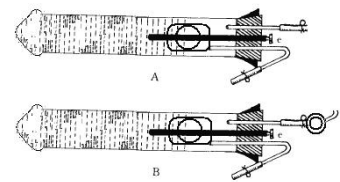
图 6 A 流动电极 B 脉冲电极
