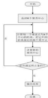
图 K-means 聚类算法流程图
