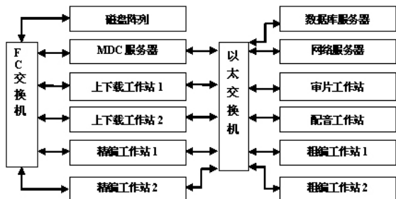
图 1 非编网络结构示意图
