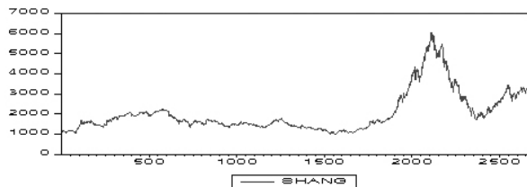
图 1 上证综指日收盘价走势图
