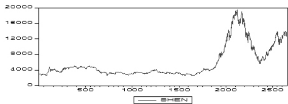
图 2 深成指日收盘价走势图
